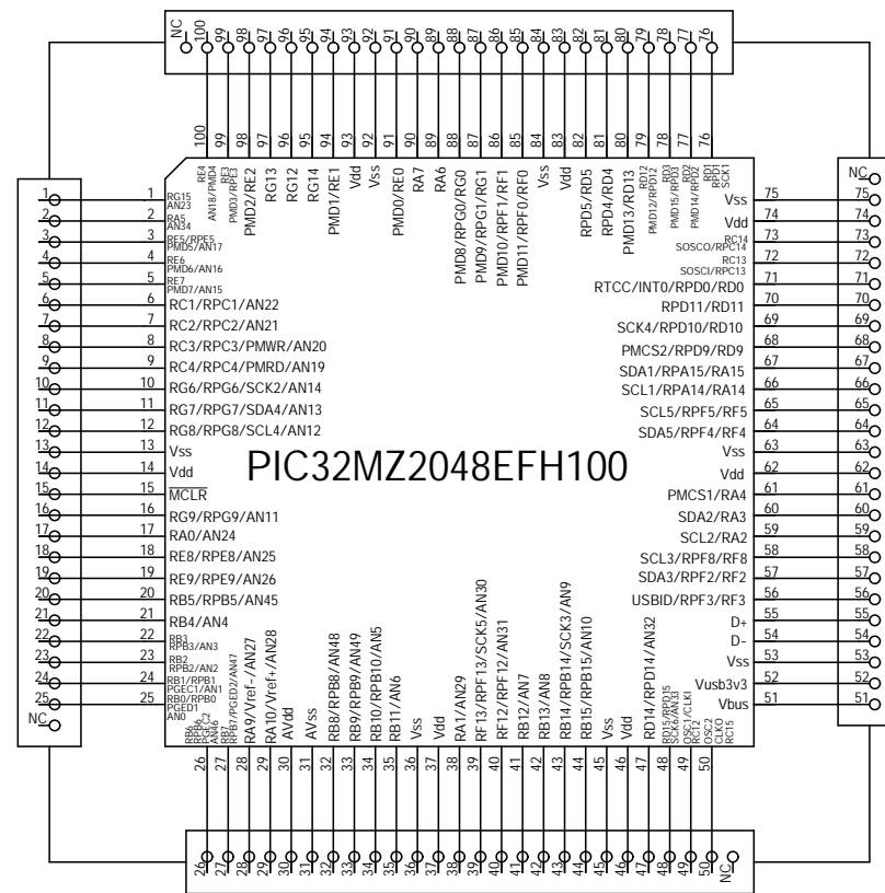
PIC32MZ2048EFH100 QFPモジュール 回路図
